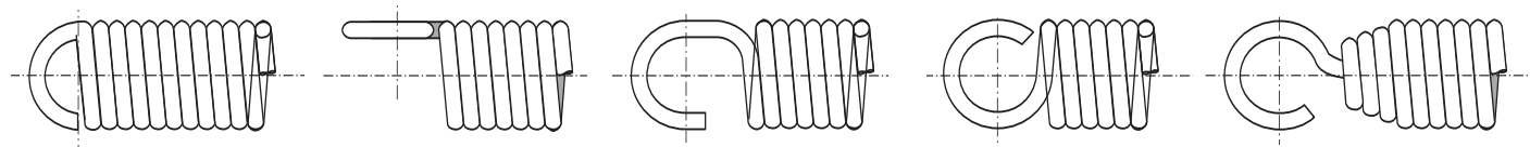
německé půl oko
