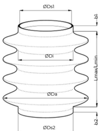
Cylindrická manžeta
