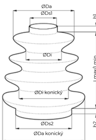
Kónická manžeta
