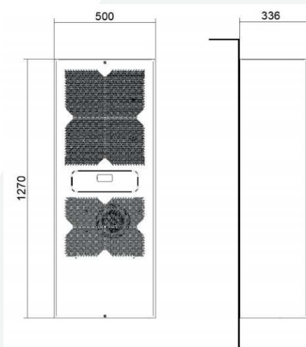
Rozměry
