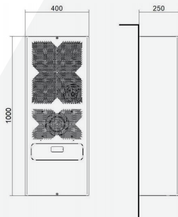
Rozměry
