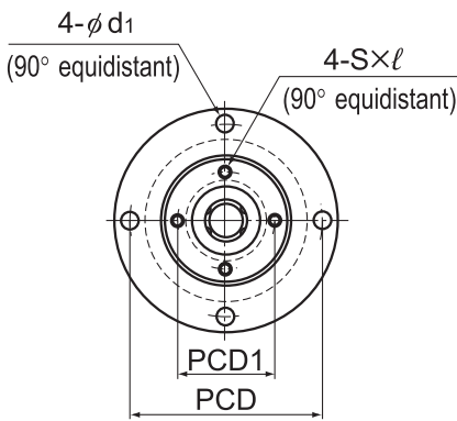
Model LTR8A Model LTR10A
