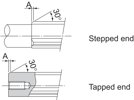
Fig. 2 Chamfer A
