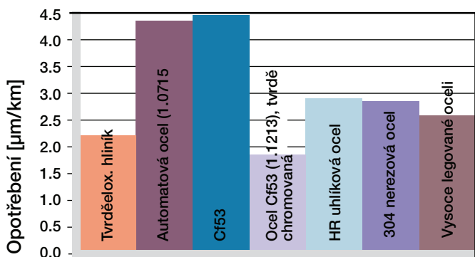
Graf 08: Opatření, rotační pohyb, tlak p = 1 MPa, v = 0,3 m/s
